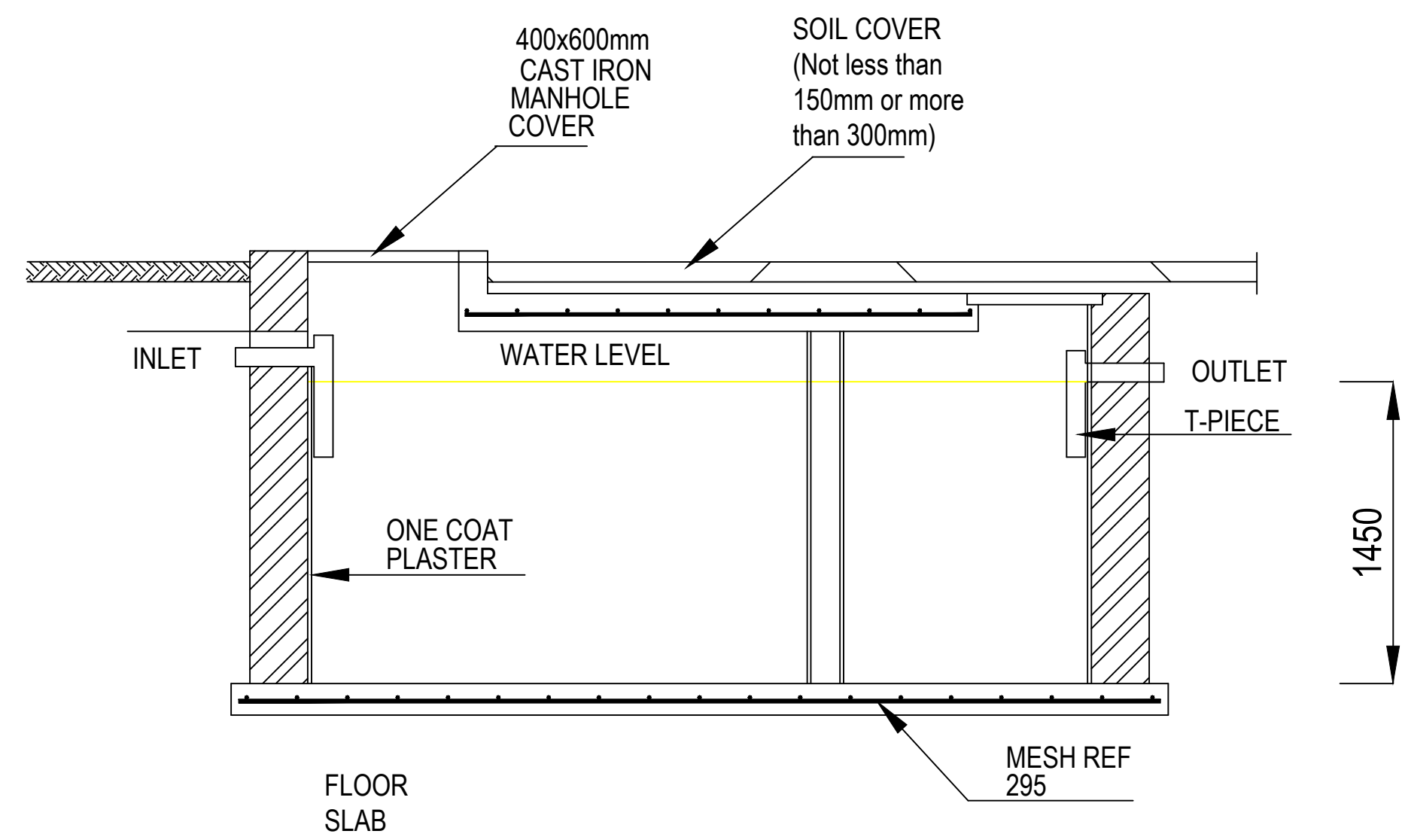
SECTION A-A
